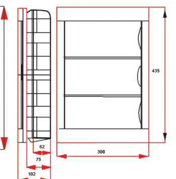
8036 внутрішній монтаж
