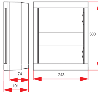
8136 зовнішній монтаж
