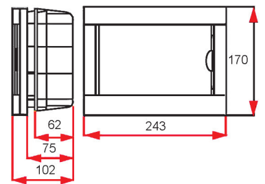
8009 внутрішній монтаж
