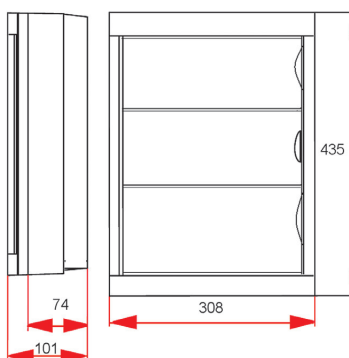
8136 зовнішній монтаж
