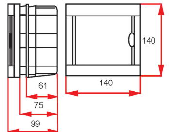
8004 внутрішній монтаж
