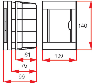
8002 внутрішній монтаж
