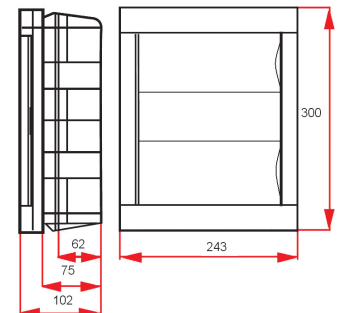
8036 внутрішній монтаж
