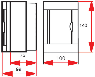
8102 зовнішній монтаж
