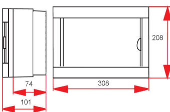
8112 зовнішній монтаж
