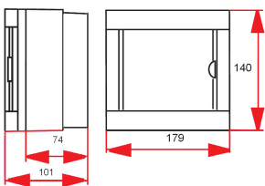
8106 зовнішній монтаж
