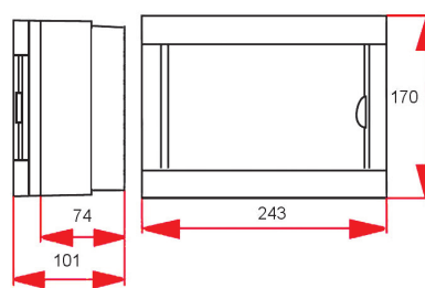
8109 зовнішній монтаж
