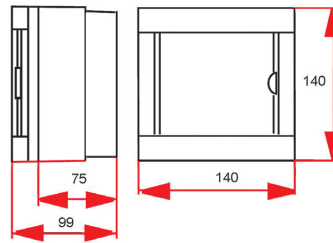
8104 зовнішній монтаж
