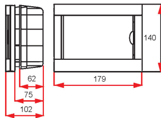
8006 внутрішній монтаж
