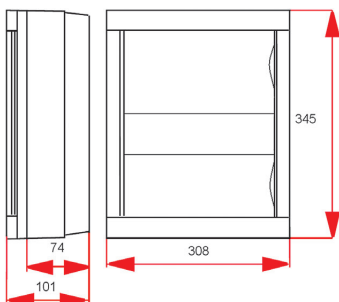
8124 зовнішній монтаж
