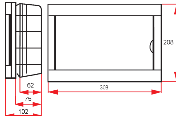
8012 внутрішній монтаж
